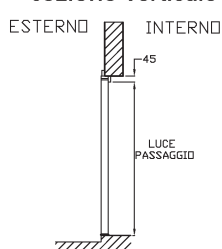
Porta con battuta inferiore sezione verticale
