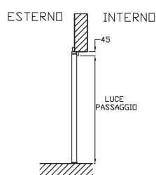
Porta senza battuta inferiore sezione verticale
